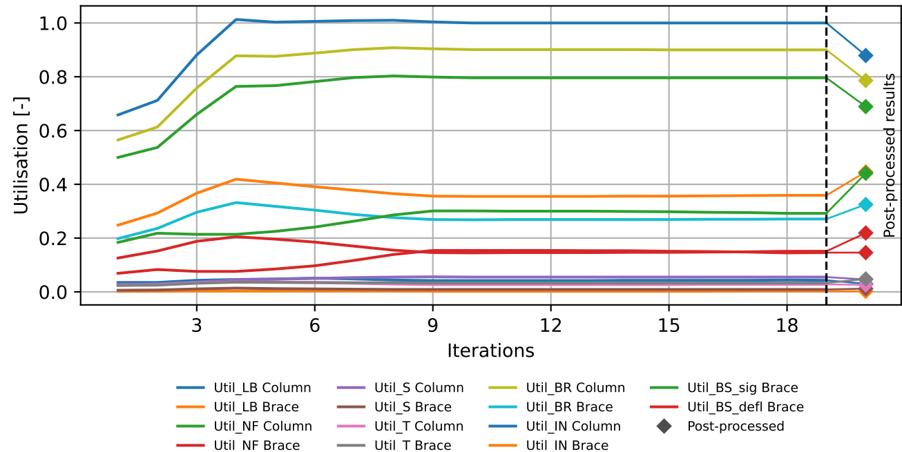
SLP Constraint utilisation history
